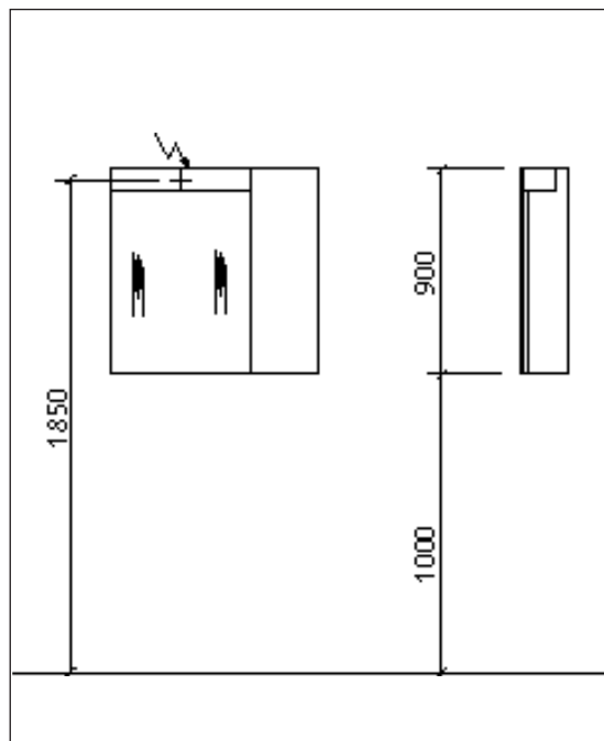
Empfohlene Montagehöhe
