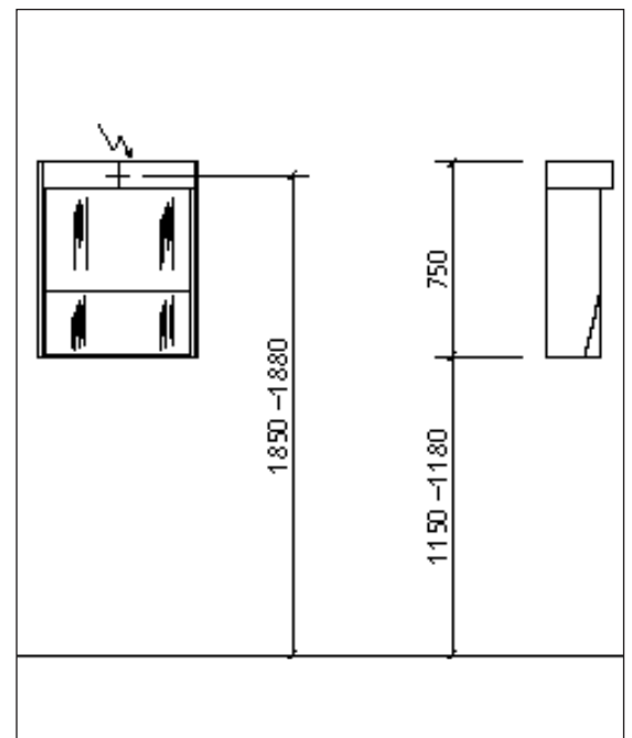
Empfohlene Montagehöhe
